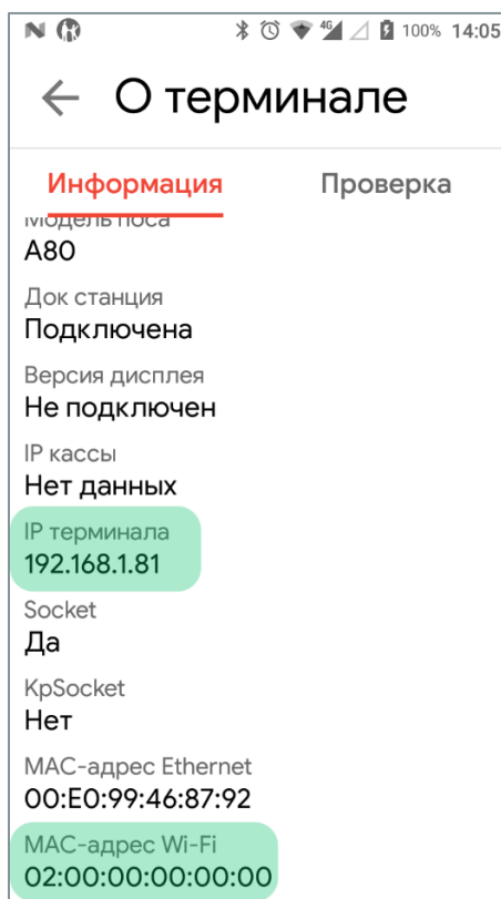
Рисунок 3.12.2.2 - Информация о закреплённом адресе
