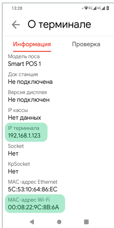
Рисунок 3.13.2.2 - Информация о закрепленном адресе
