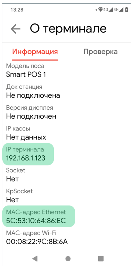
Рисунок 3.13.1.3 – Информация о закрепленном адресе
