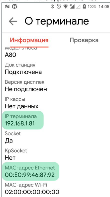
Рисунок 3.12.1.3 – Информация о закрепленном адресе
